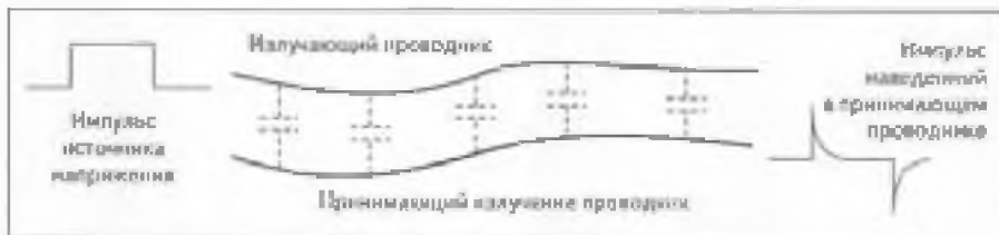
Рисунок 2 - Импульсная наводка через емкостную связь между проводниками
