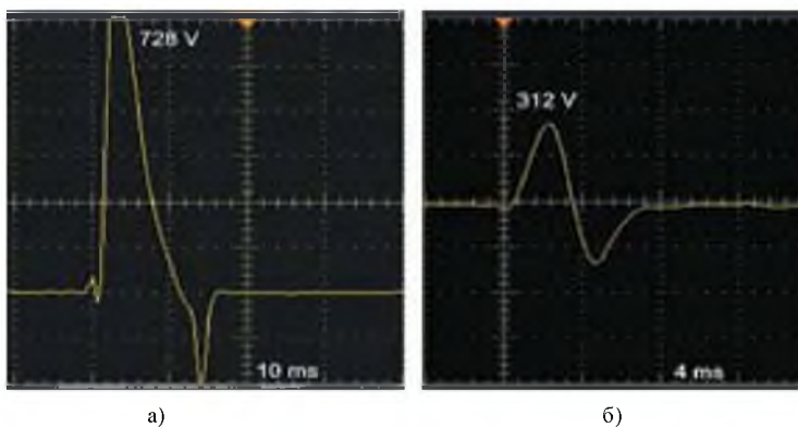
Рисунок 3 - Индуцированные наводки одного контрольного кабеля на другой
